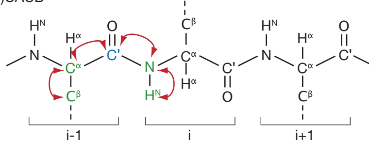
(f) HN(CO)CACB
