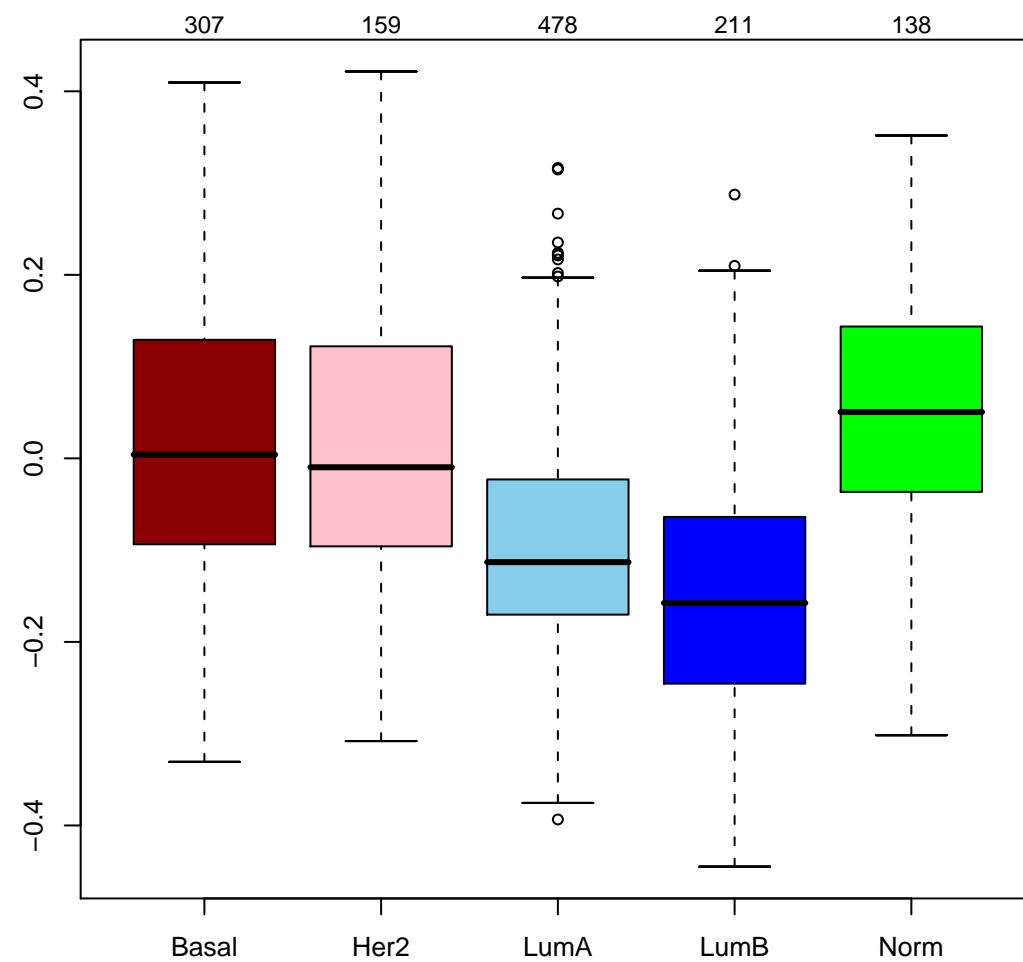
EGFR -pearson
