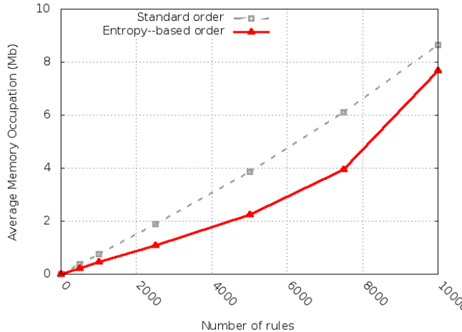
Fig. 6. JA vs Entropy-based JA
