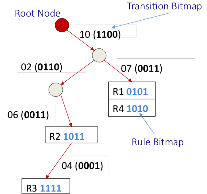
Fig. 1. JA-Trie example
